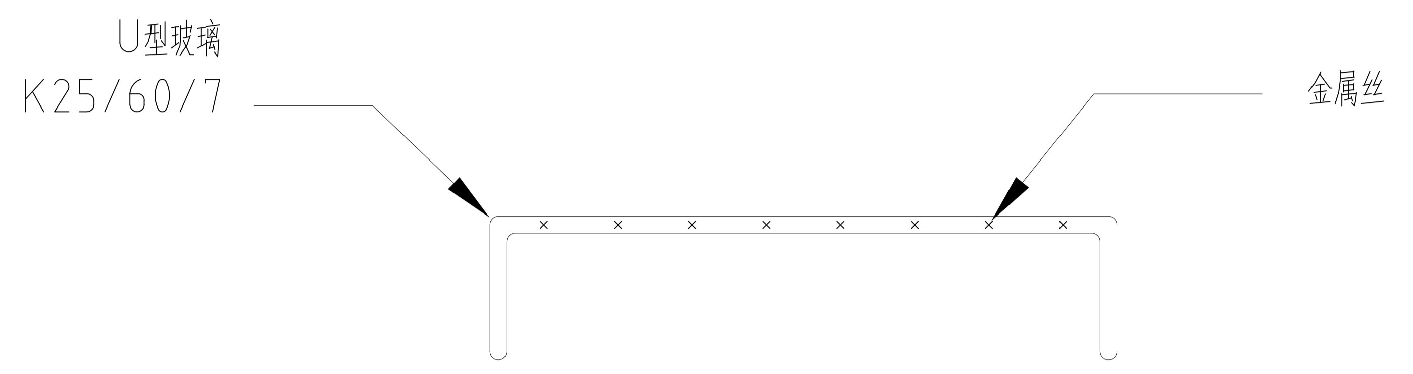
截面图
